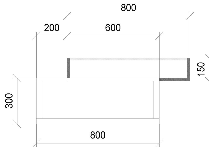
konf.stolek narys 2
