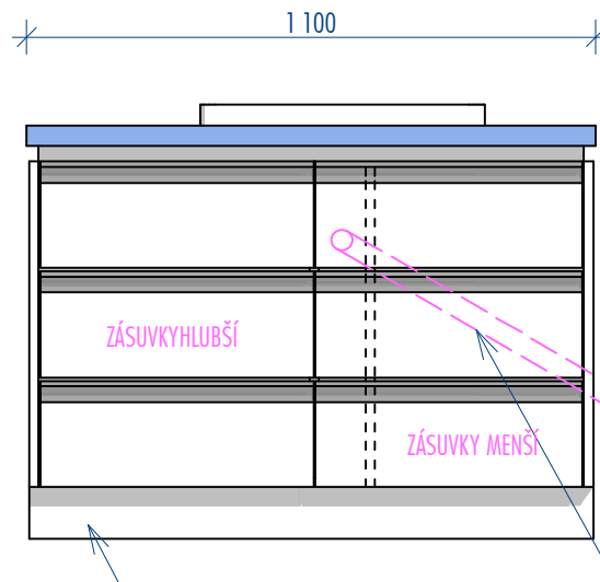
ČELNÍ POHLED
