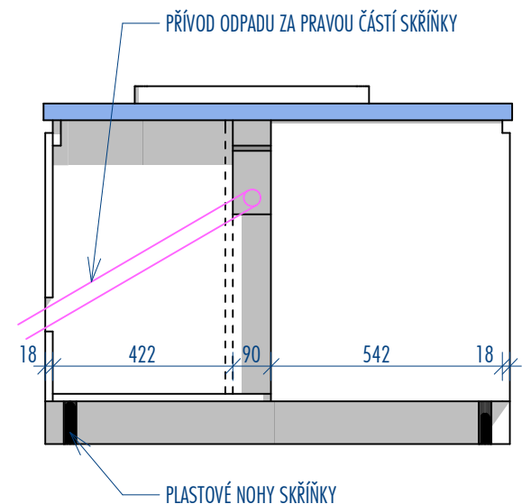
ZADNÍ POHLED
