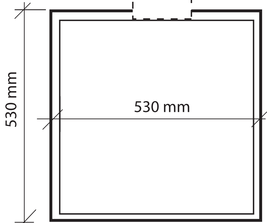
Půdorys
