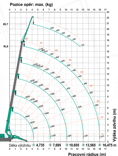
Diagram pracovní oblasti znázorňuje celkovou jmenovitou zátěž včetně dosahu výložníku.
