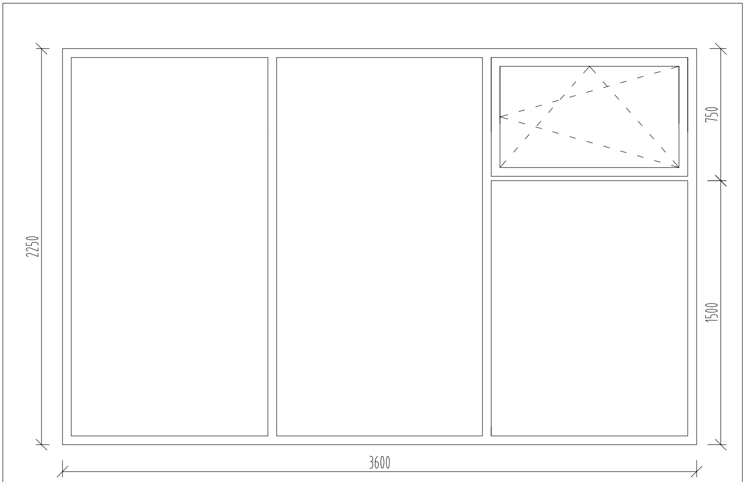
14. Okno AL. farb. antracit počet 1ks
