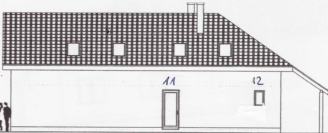
POHĽAD BOČNÝ
