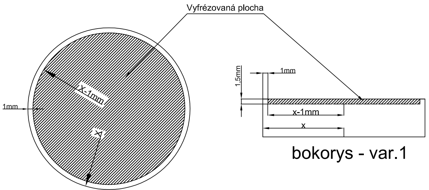
půdorys
