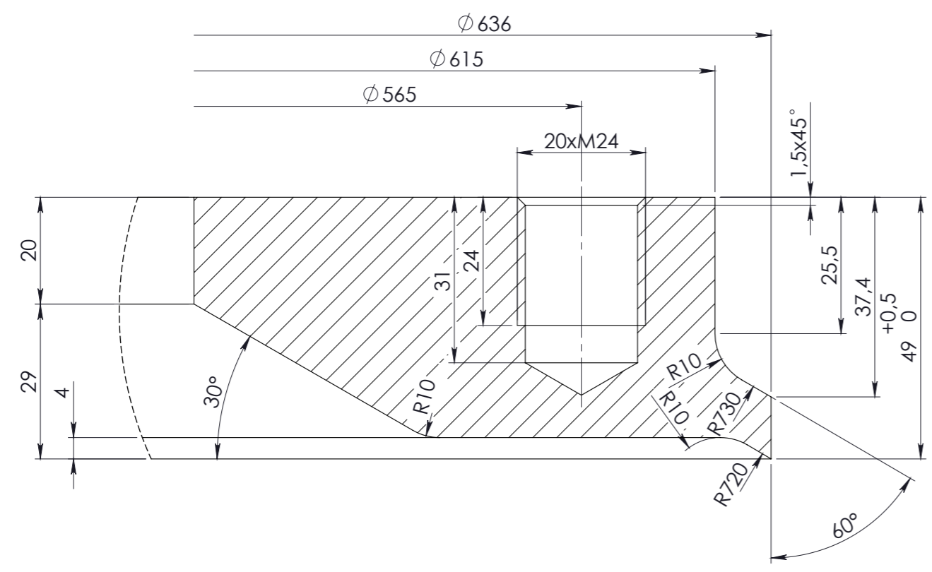
DETAIL B MĚŘITKO 1 : 1
