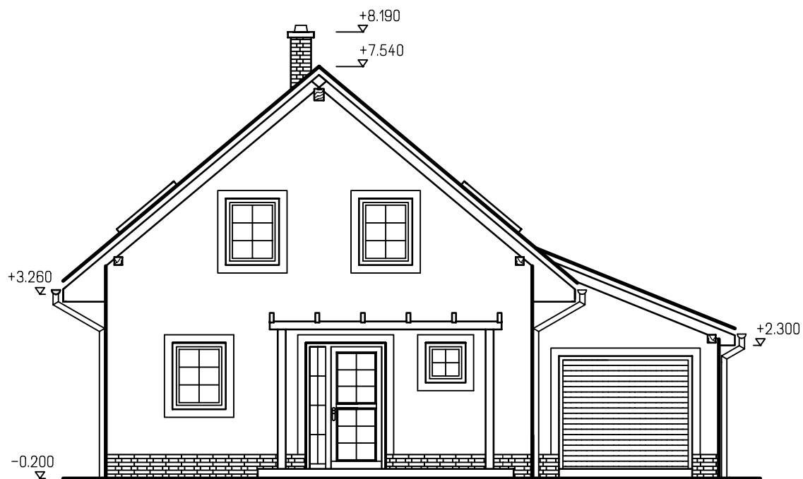
POHLED ČELNÍ
