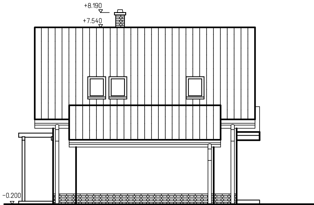
POHLED BOČNÍ
