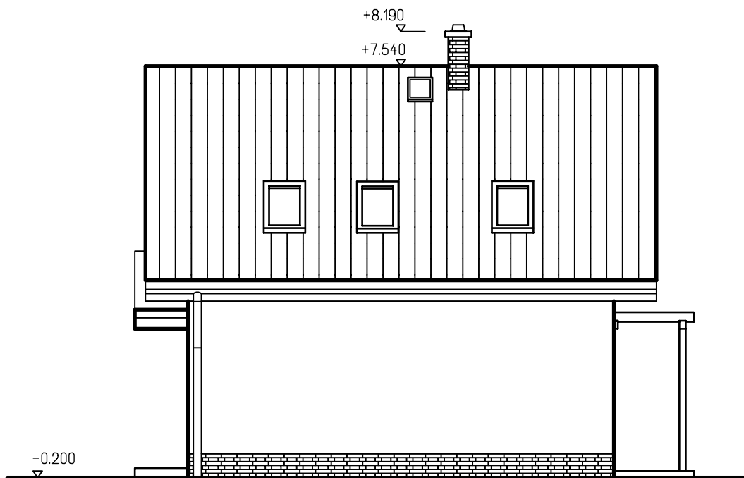
POHLED BOČNÍ
