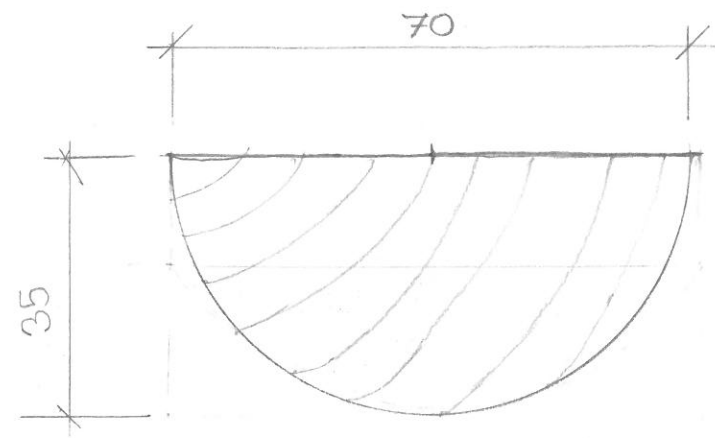
DETAIL PLANKY 1:1
