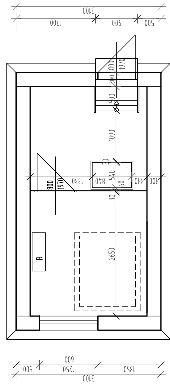
PODORYS
