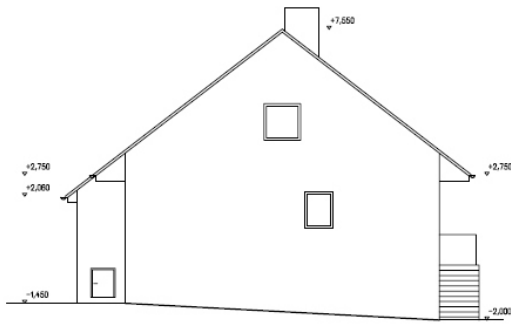
POHLED ZÁPADNÍ
