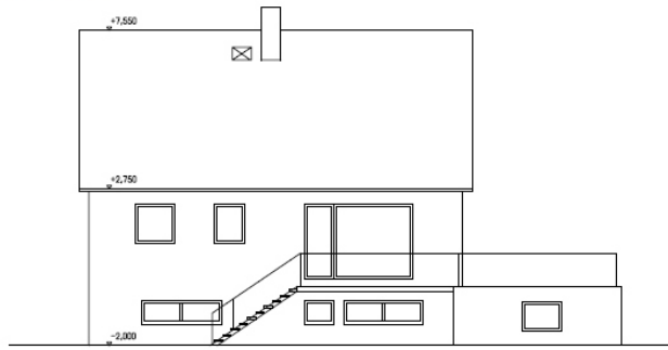
POHLED JIŽNÍ
