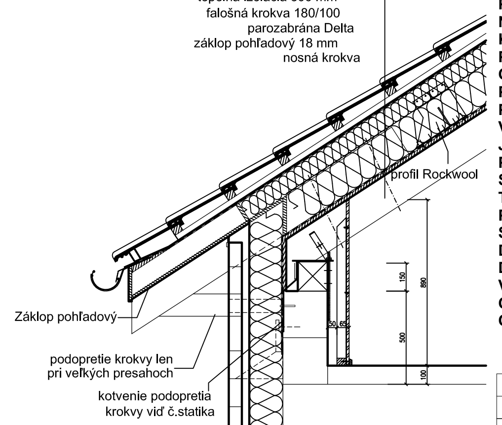
Strešný plášť 1 : 20
