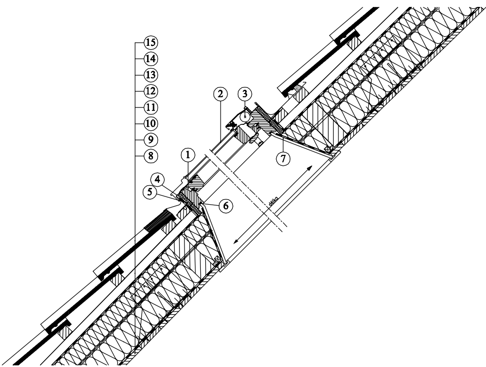
Strešný plášť 1 : 20
