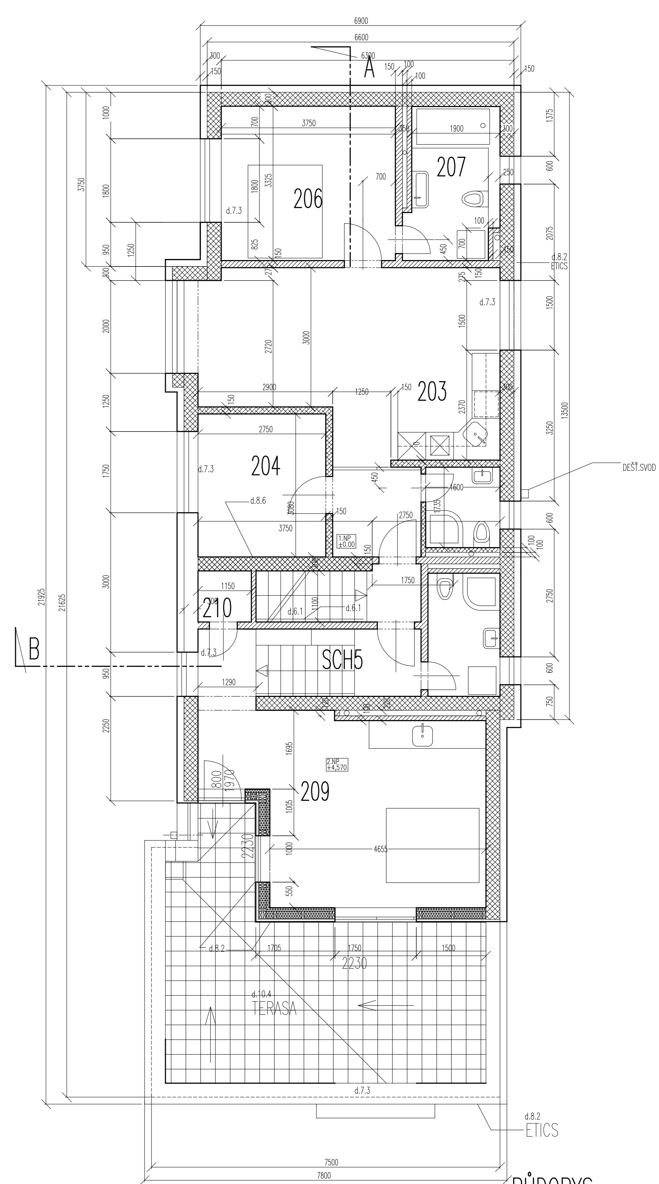
PŮDORYS 2.NP
