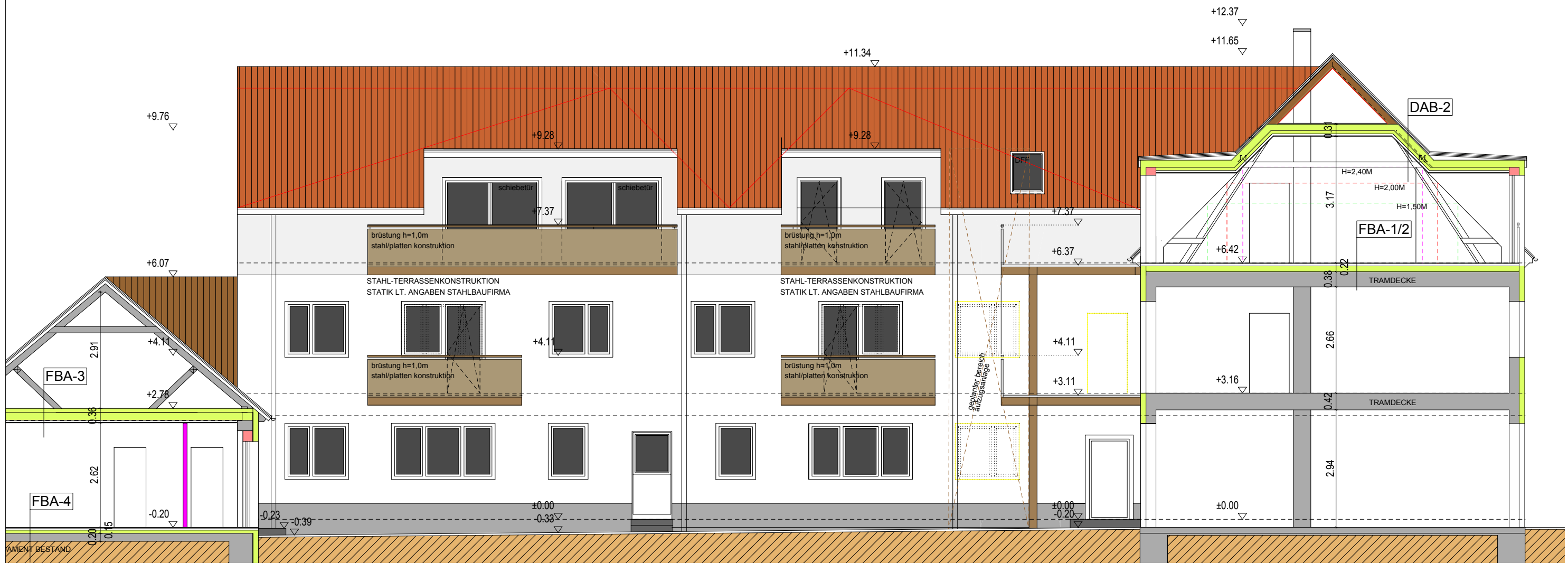
ANSICHT OST / SCHNITT C-C
