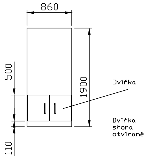
Skříň č.6 hl. 330mm
