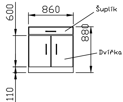
Skříňka č.8 hl. 330mm
