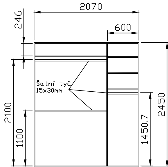
Skříň č.4 hl. 540mm
