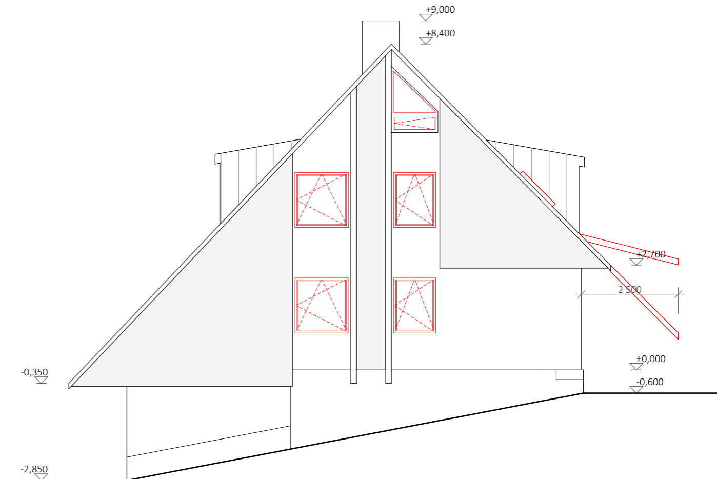
POHLED JIHOVÝCHODNÍ
