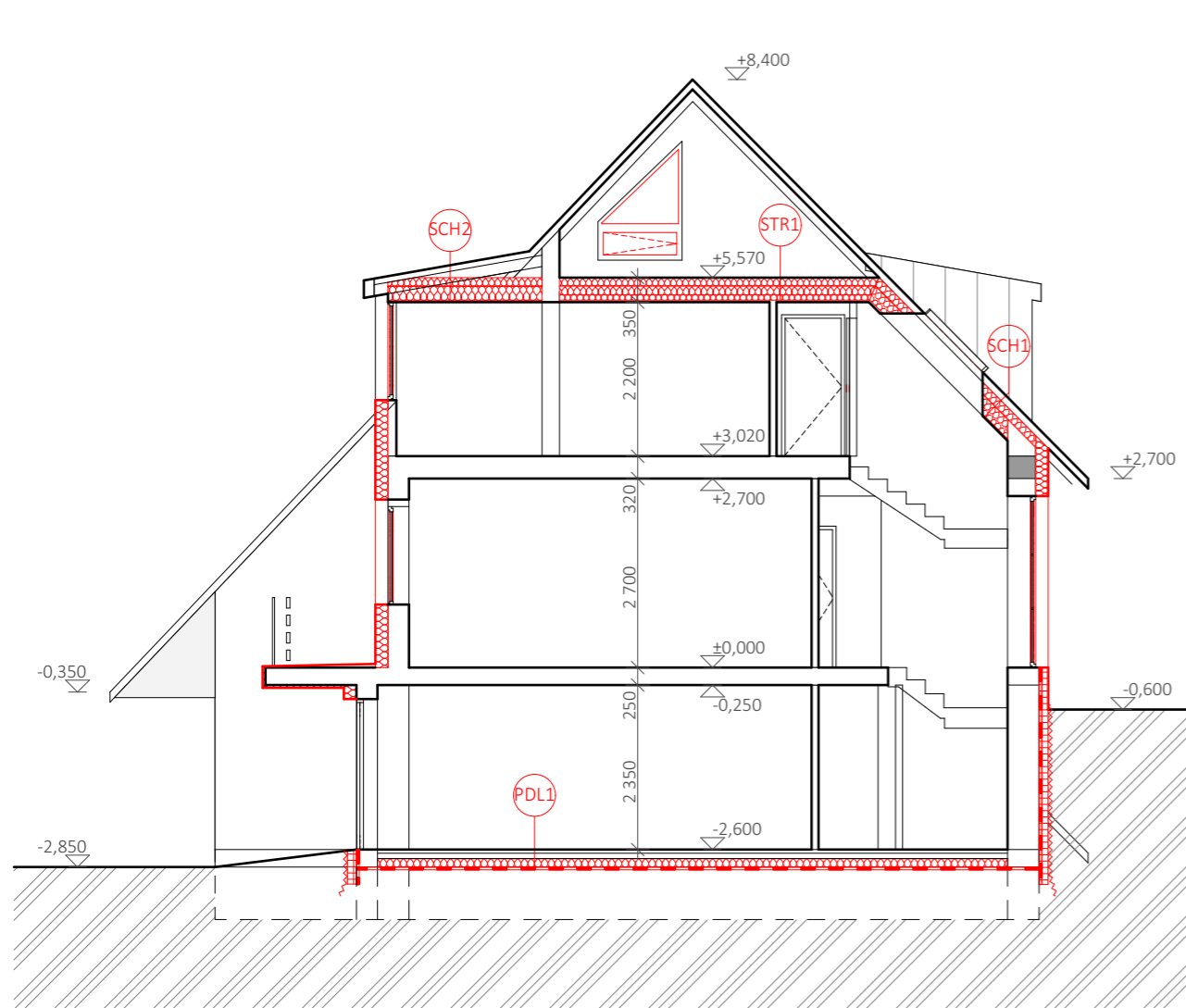
ŘEZ A-A
