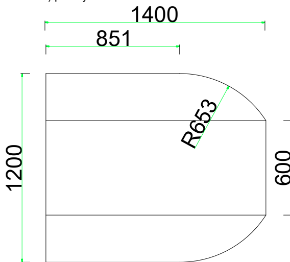
a) půdorys
