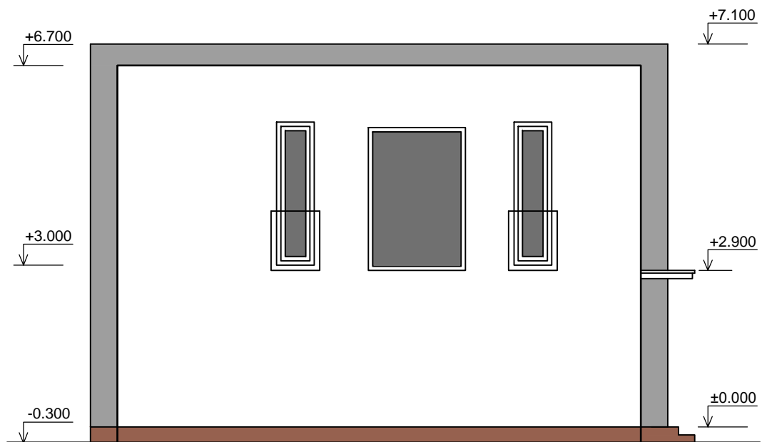
POHLED SEVEROVÝCHODNÍ - M 1:100
