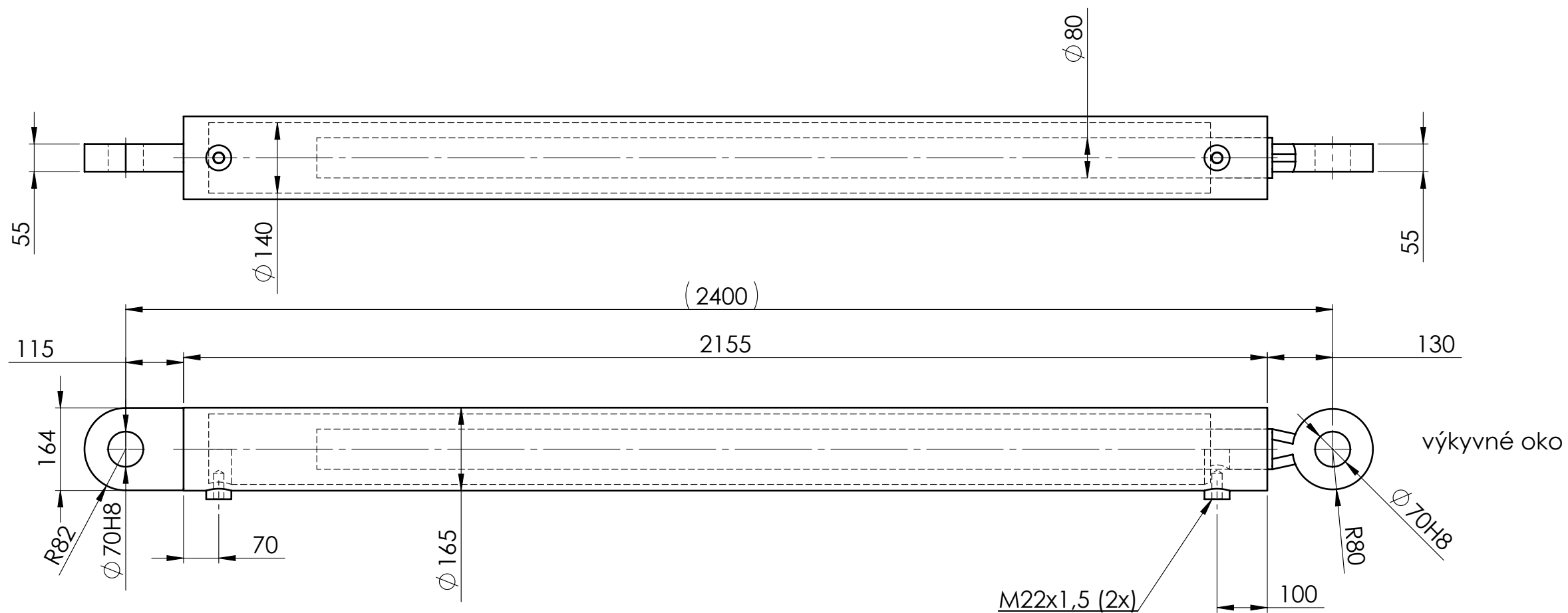
Píst 140/80/1900 počet kusů 2
