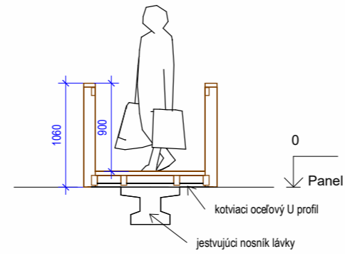
Priečny rez AA 1:50
