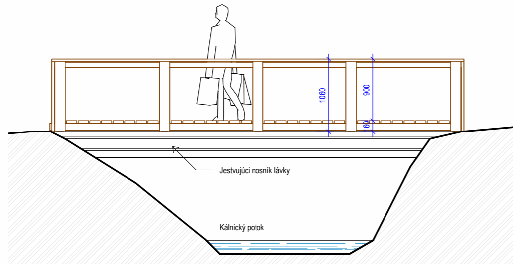
Rezopohľad BB 1:50
