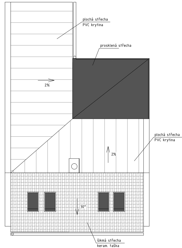
STŘECHA
