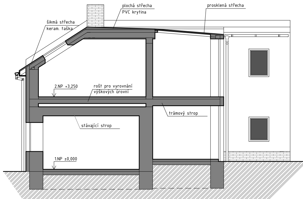
POHLED DVORNÍ/ŘEZ
