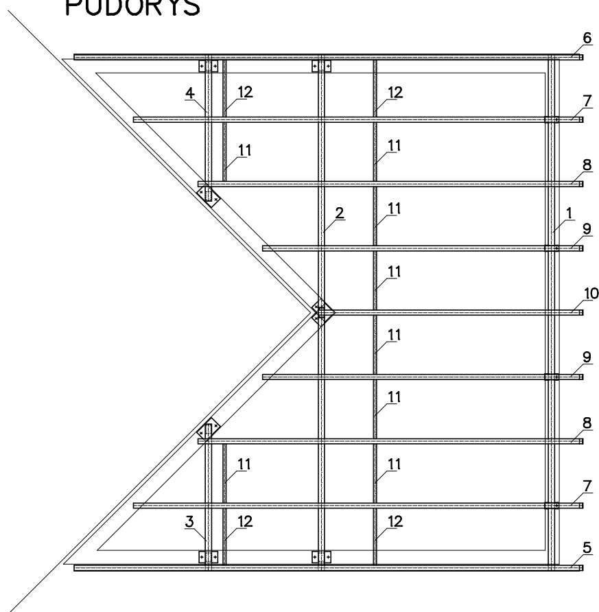
PŮDORYS
