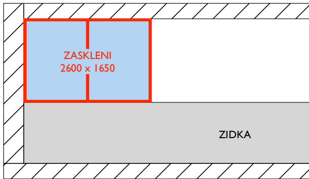
Pohled A
