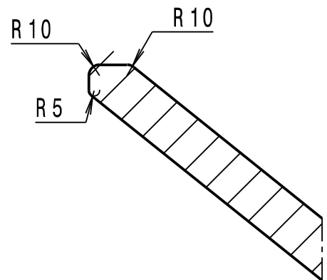
REZ D-D MIERKA 1:5
