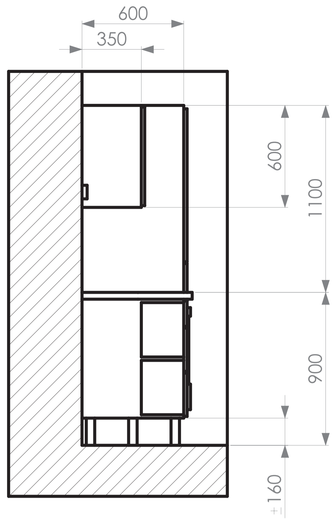
ŘEZ D-D
