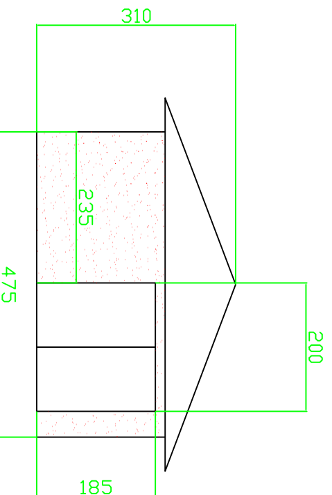
PŮDORYS+ KROKVE
