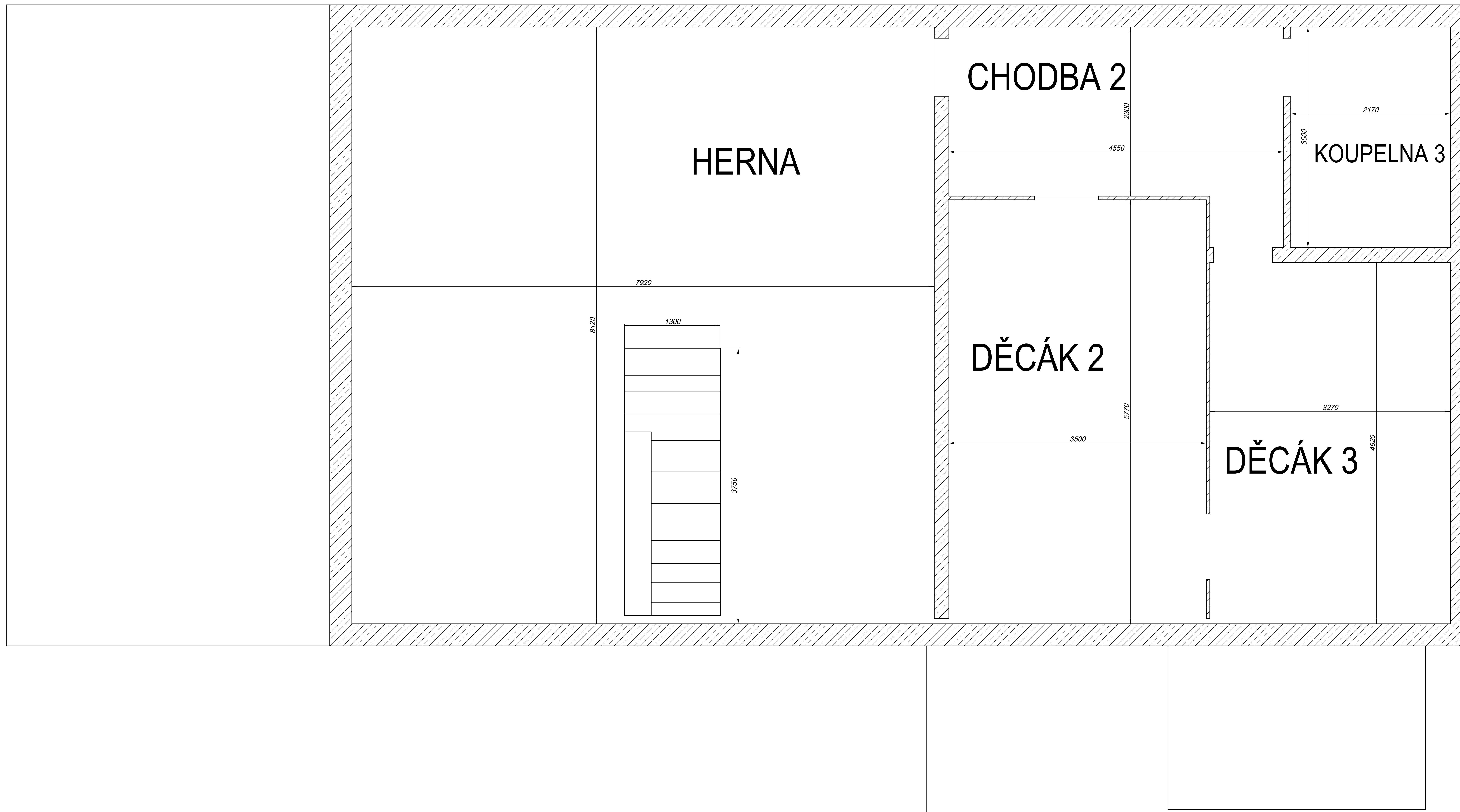
B-B (1 : 20)
