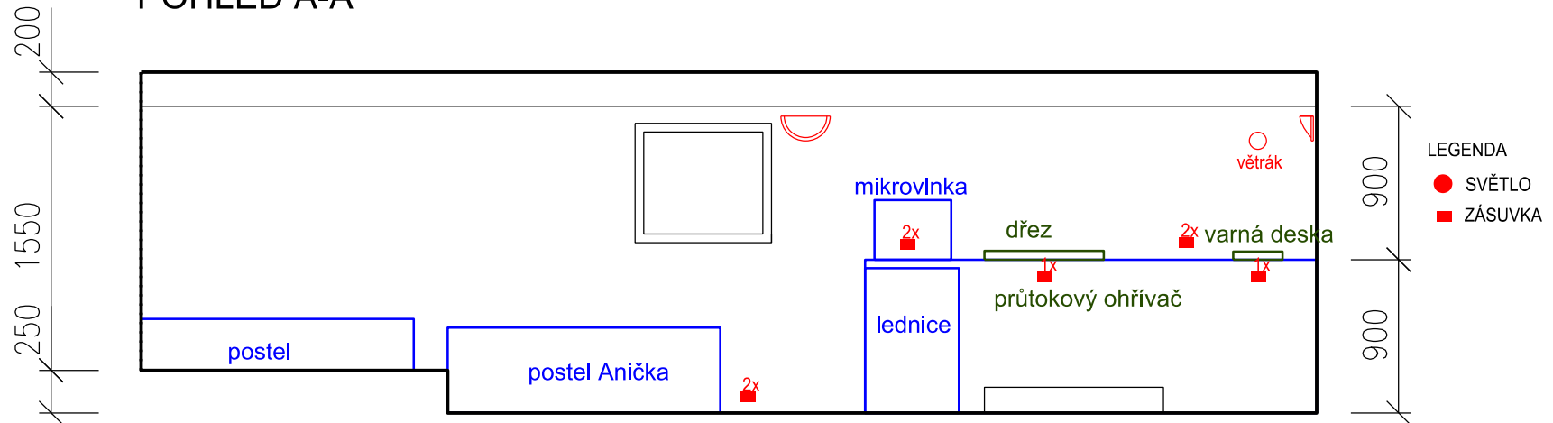
POHLED A-A
