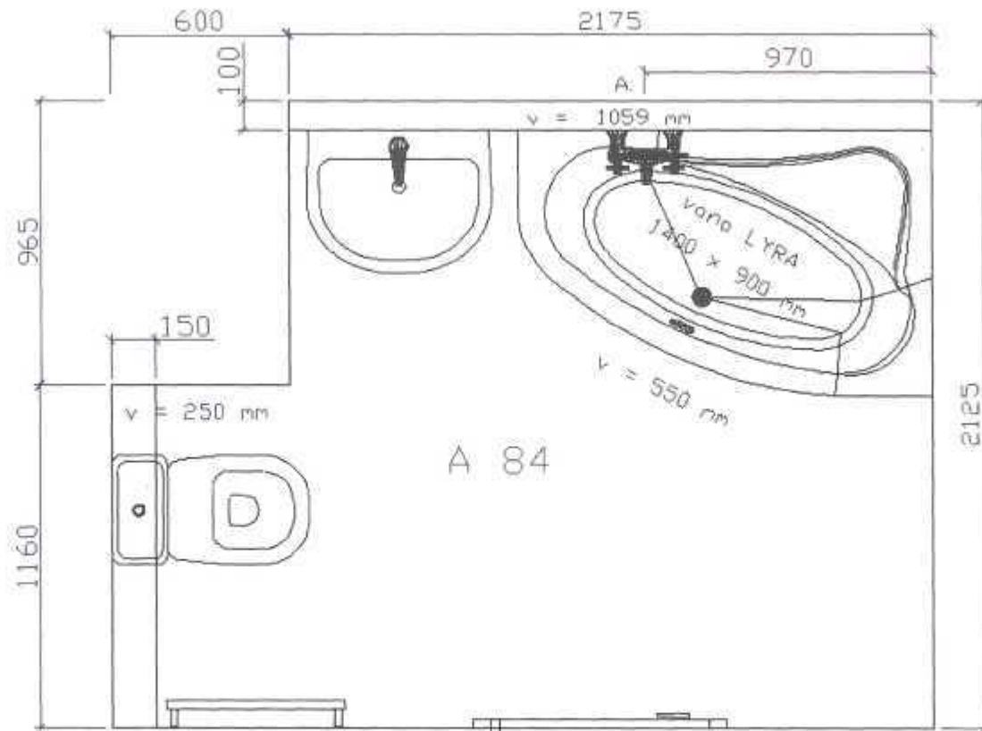
koupelna pôdorys (826x670x16M jpeg)
