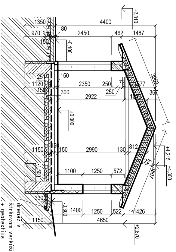
REZ B-B
