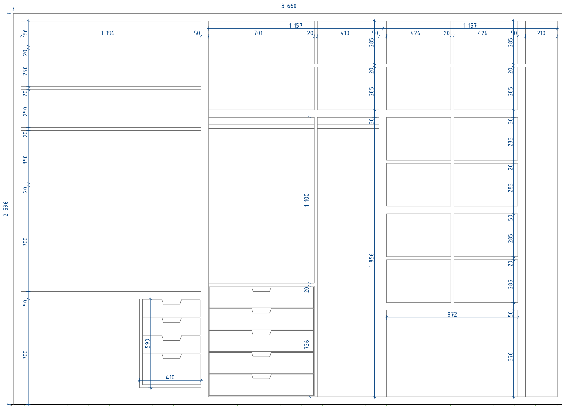
Vestavěná skříň s pracovním stolem - obývací pokoj, hloubka skříně 650 mm, M 1:15
