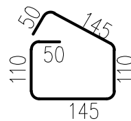
∅ R 6 – 0,61 m 10 ks
