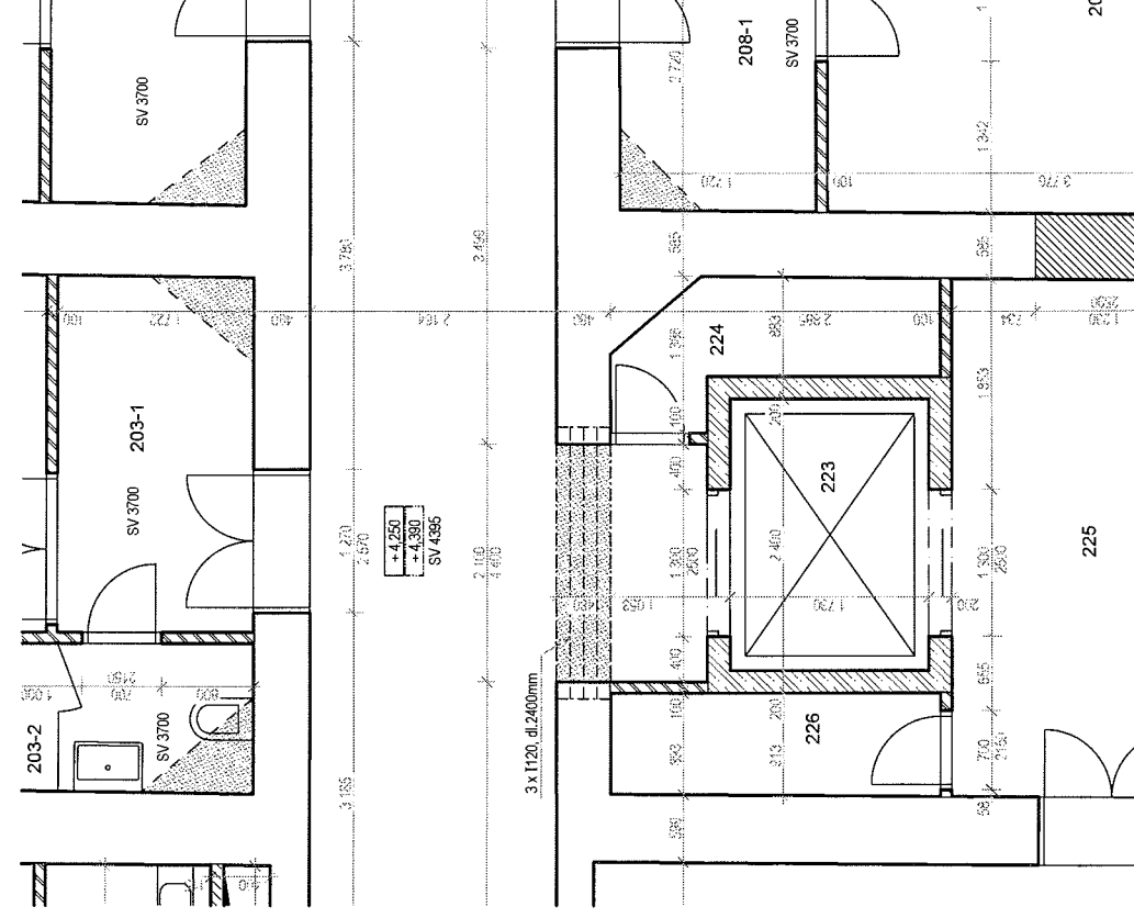
PŮDORYS 2.NADZEMNÍHO PODLAŽÍ
