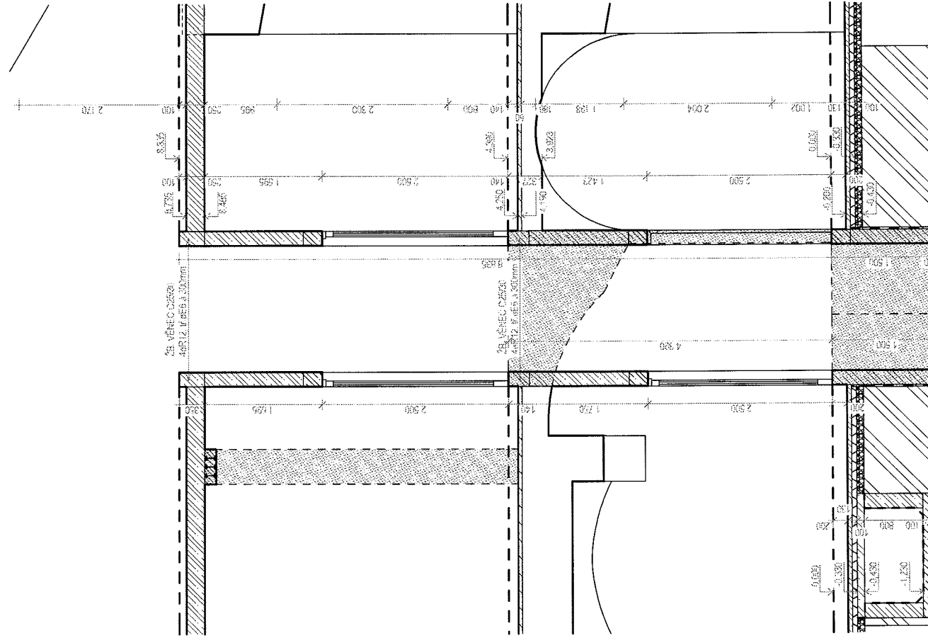
ŘEZ VÝTAHOVOU ŠACHTOU
