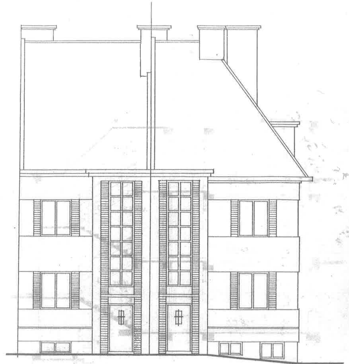
POHLED Z ULICE.
