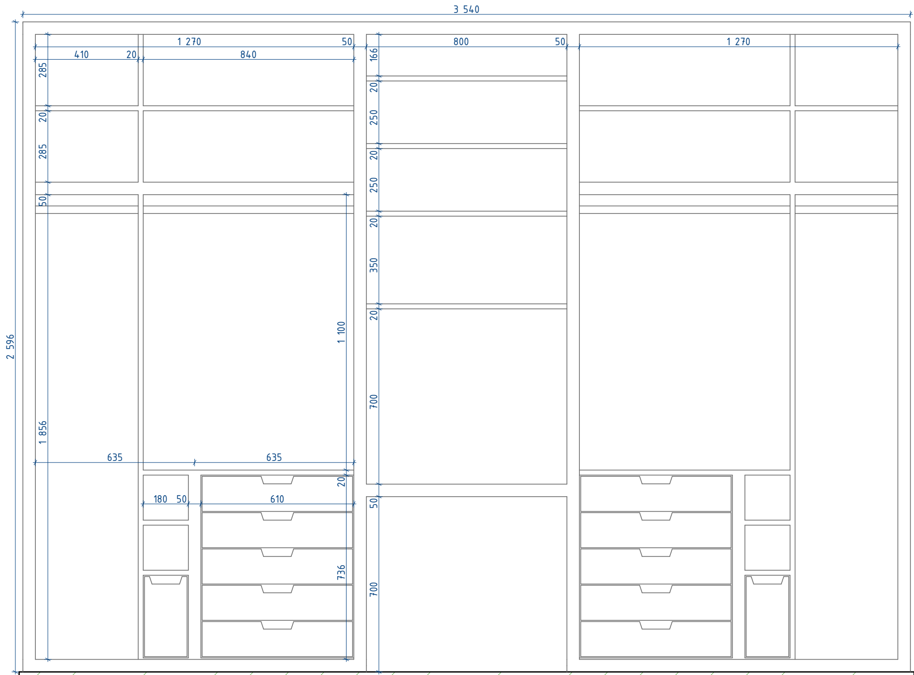
Vestavěná skříň s pracovním stolem - ložnice, hloubka skříně 650 mm, M 1:15
