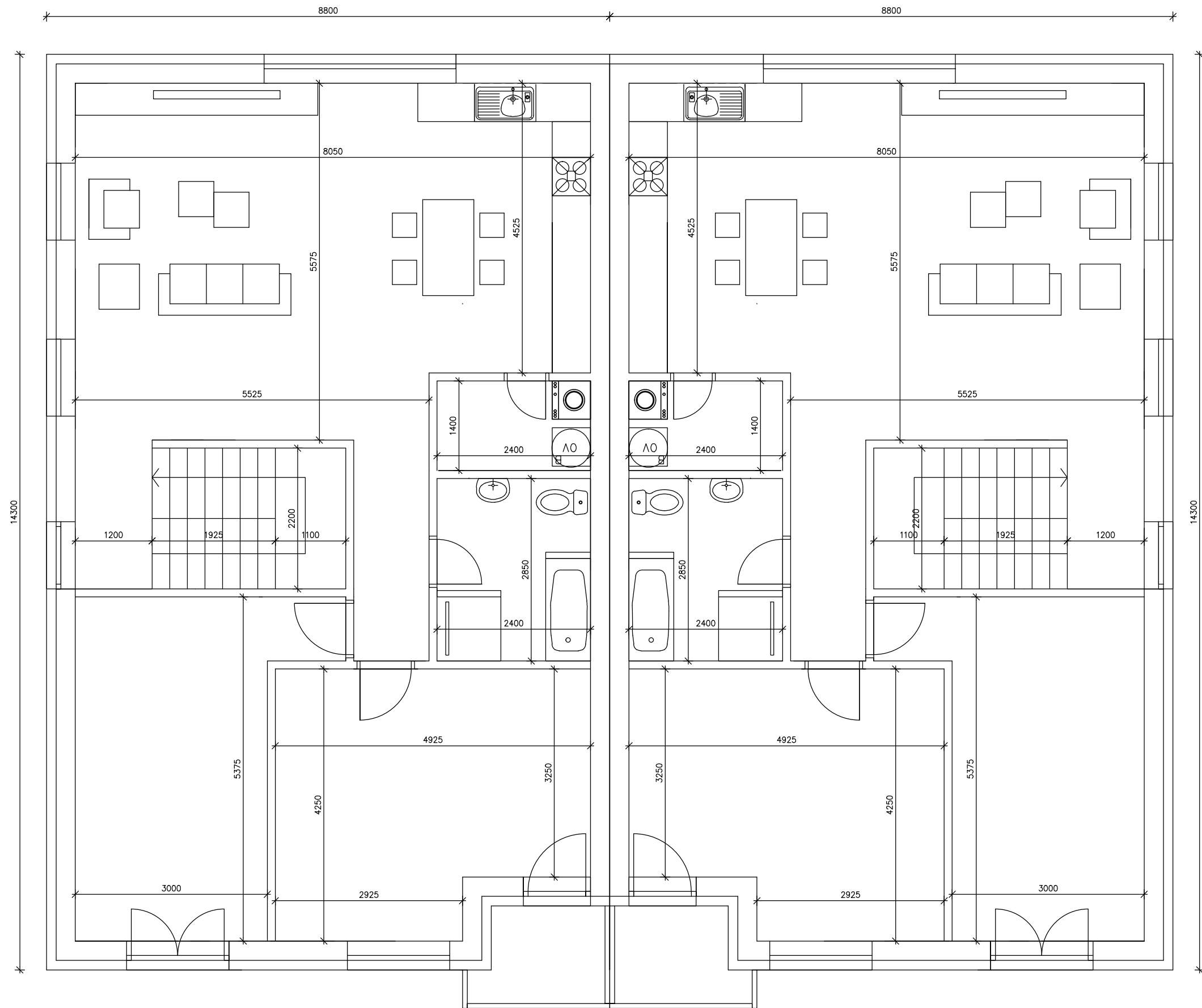
PÔDORYS POSCHODIA
