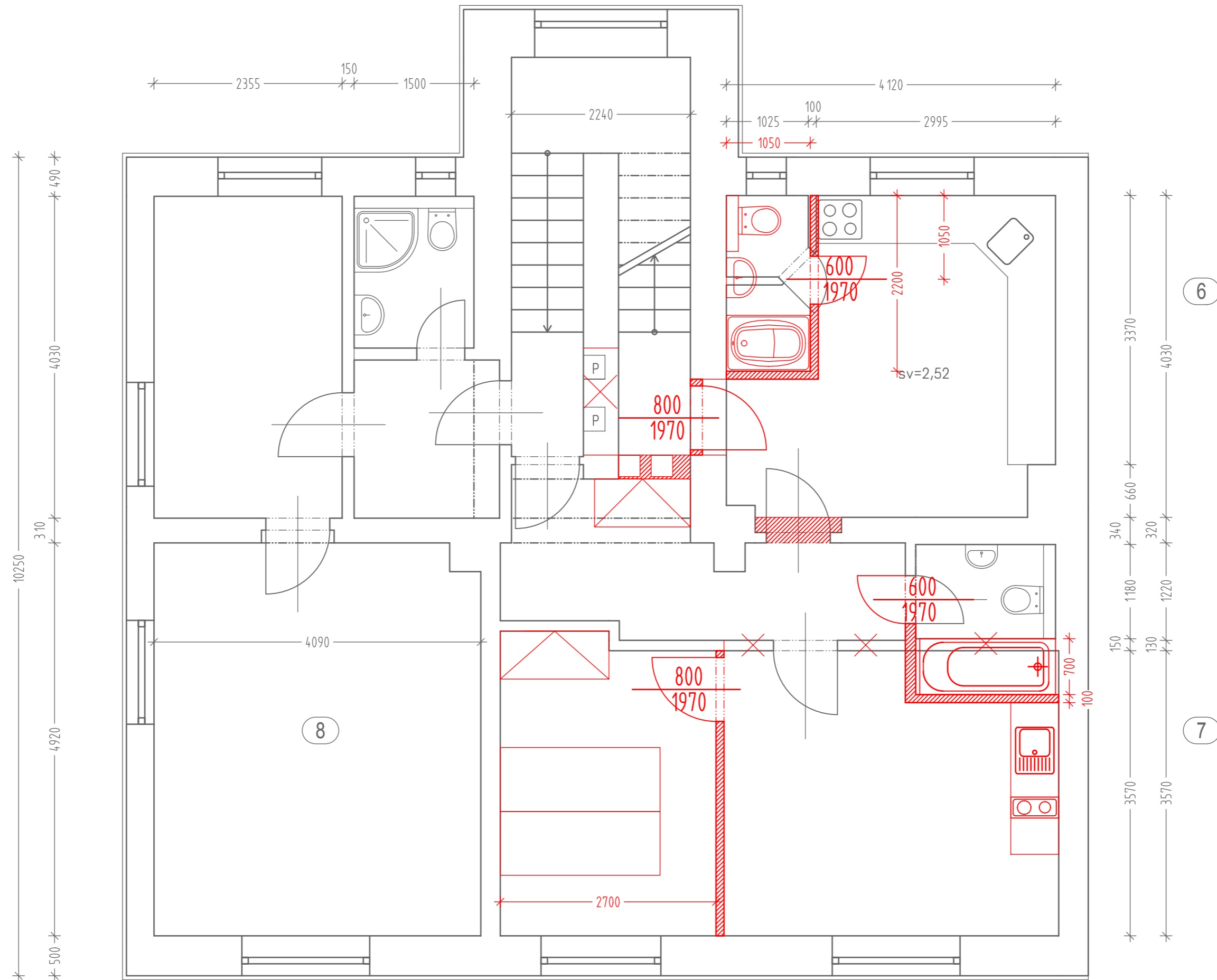
ZÁKRES DO 1.PATRA VARIANTA - a)
