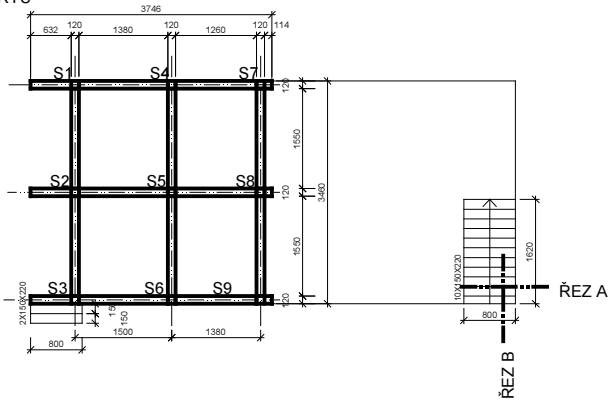
PŮDORYS
