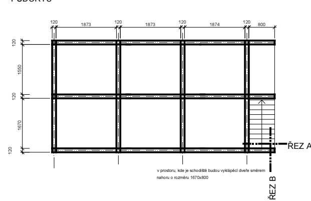
PŮDORYS
