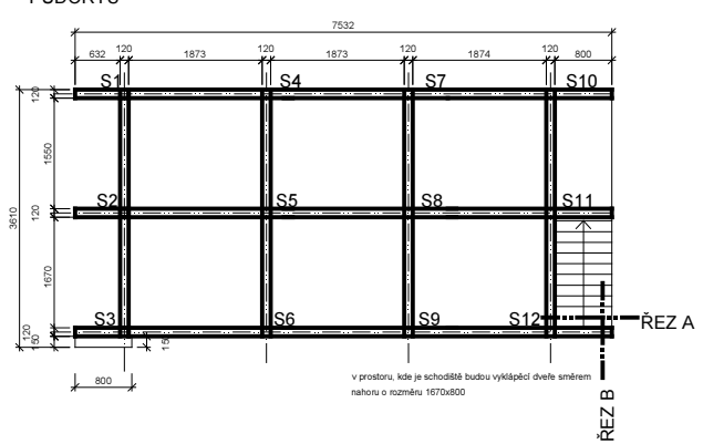
PŮDORYS
