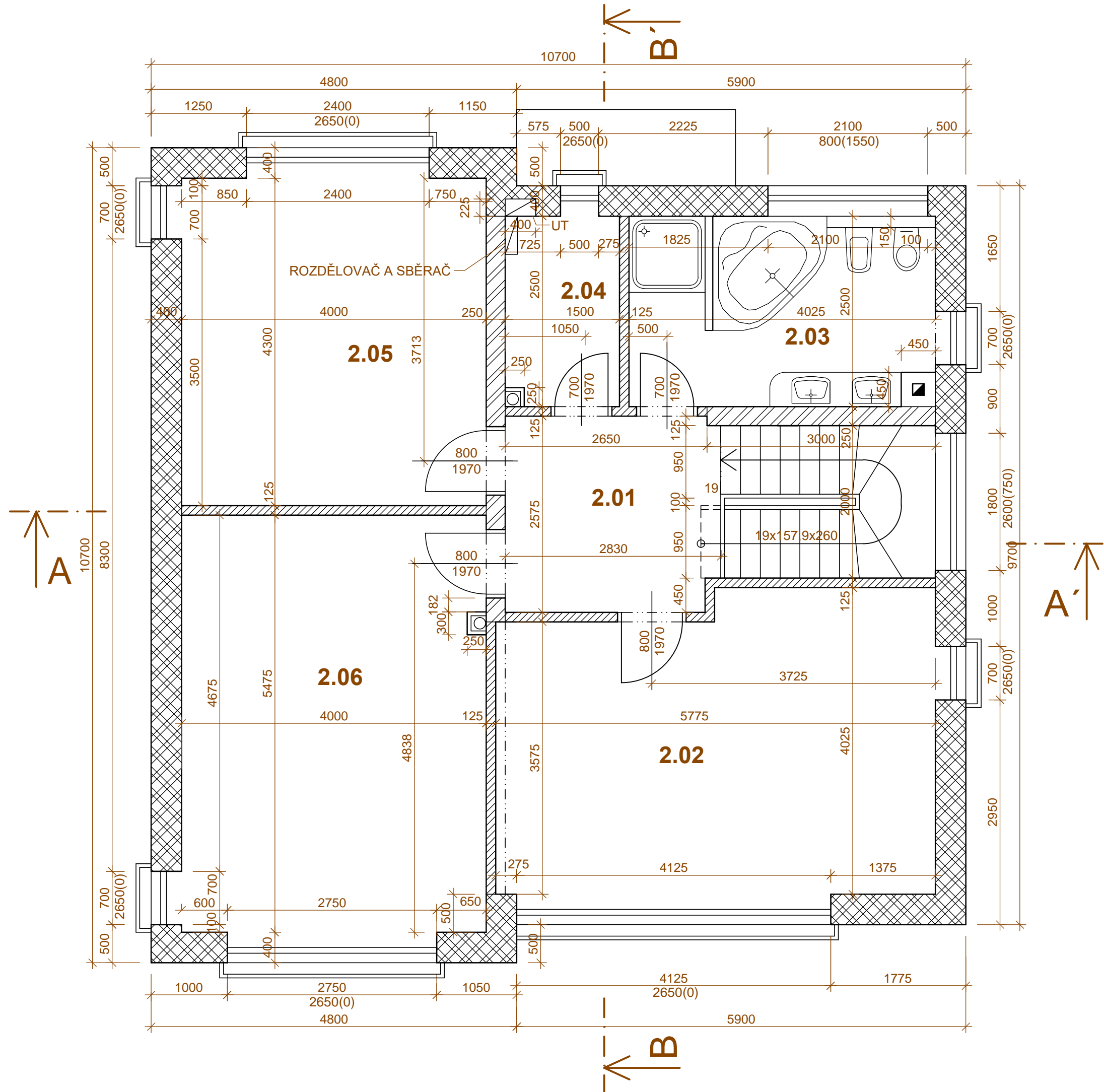
PŮDORYS 1. PATRA - M 1:50
