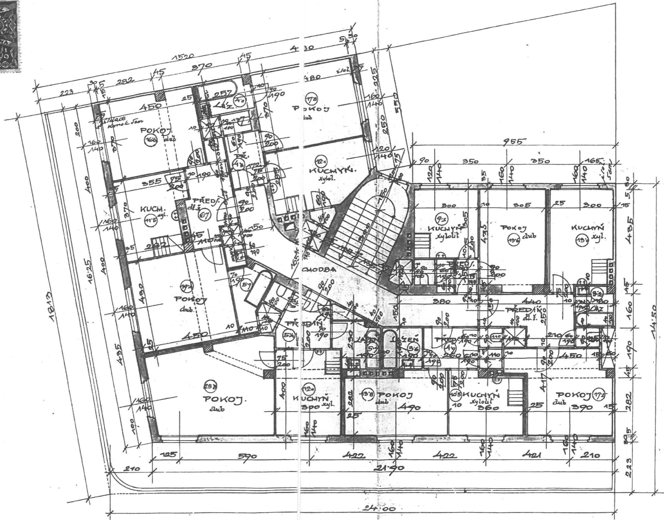
ПОДКРОВ / 1:100.
