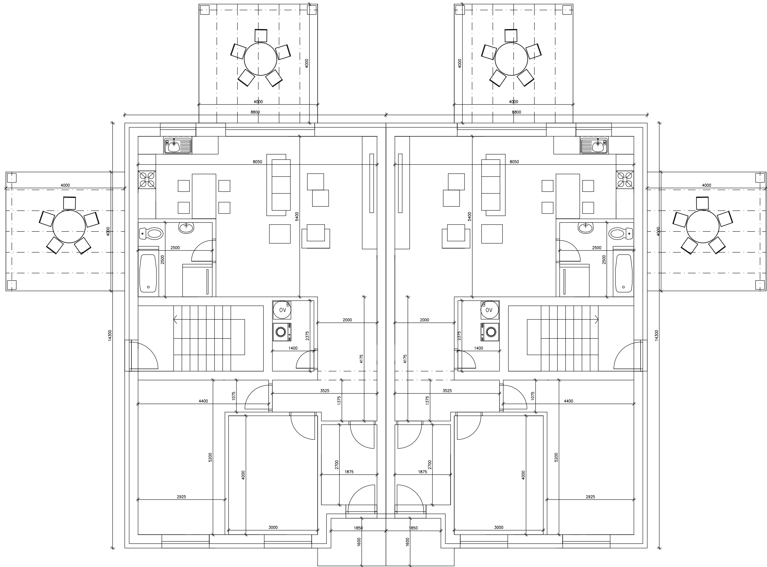
PÔDORYS PRÍZEMIA
