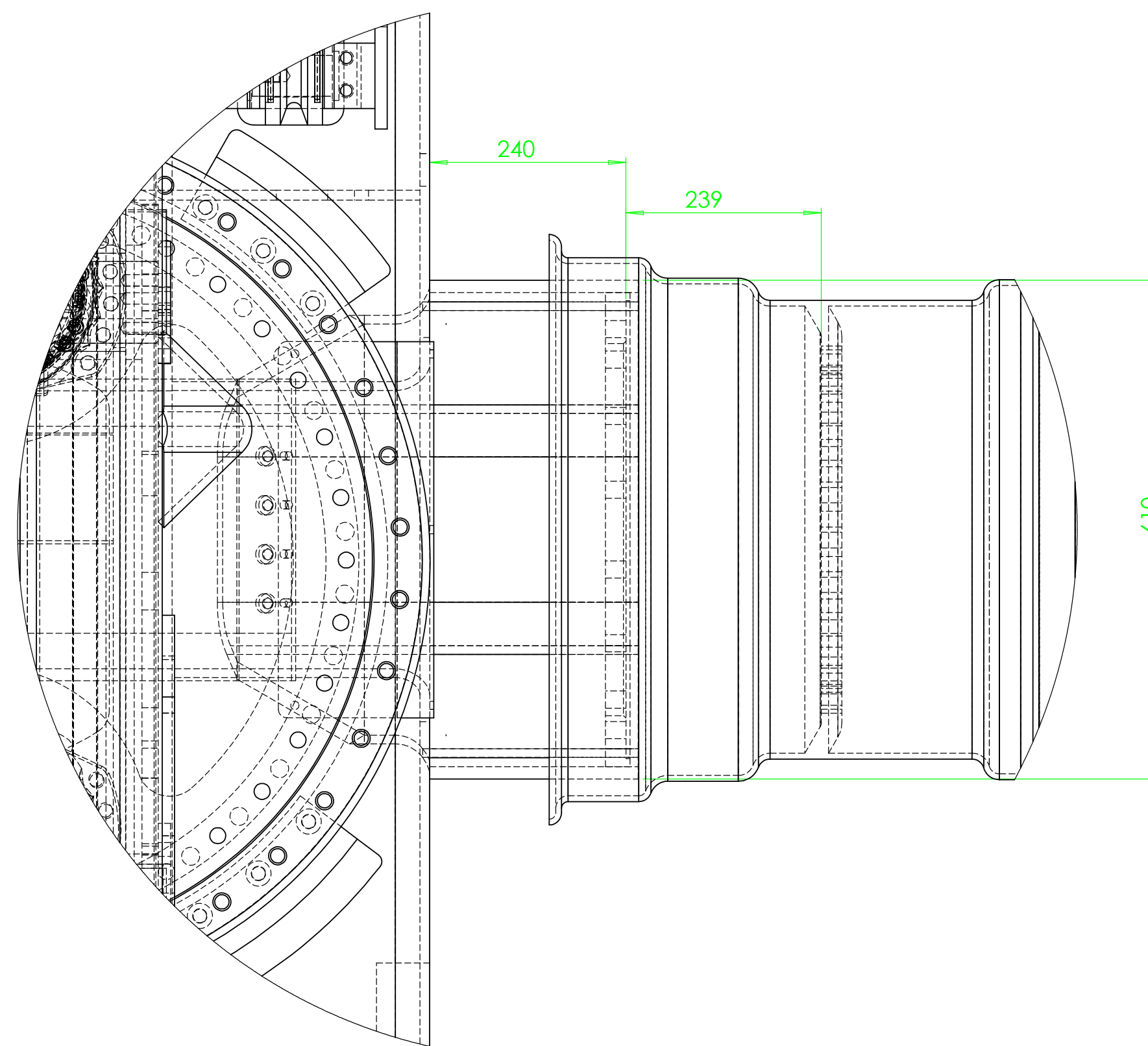
DÉTAIL A Echelle 1:6
