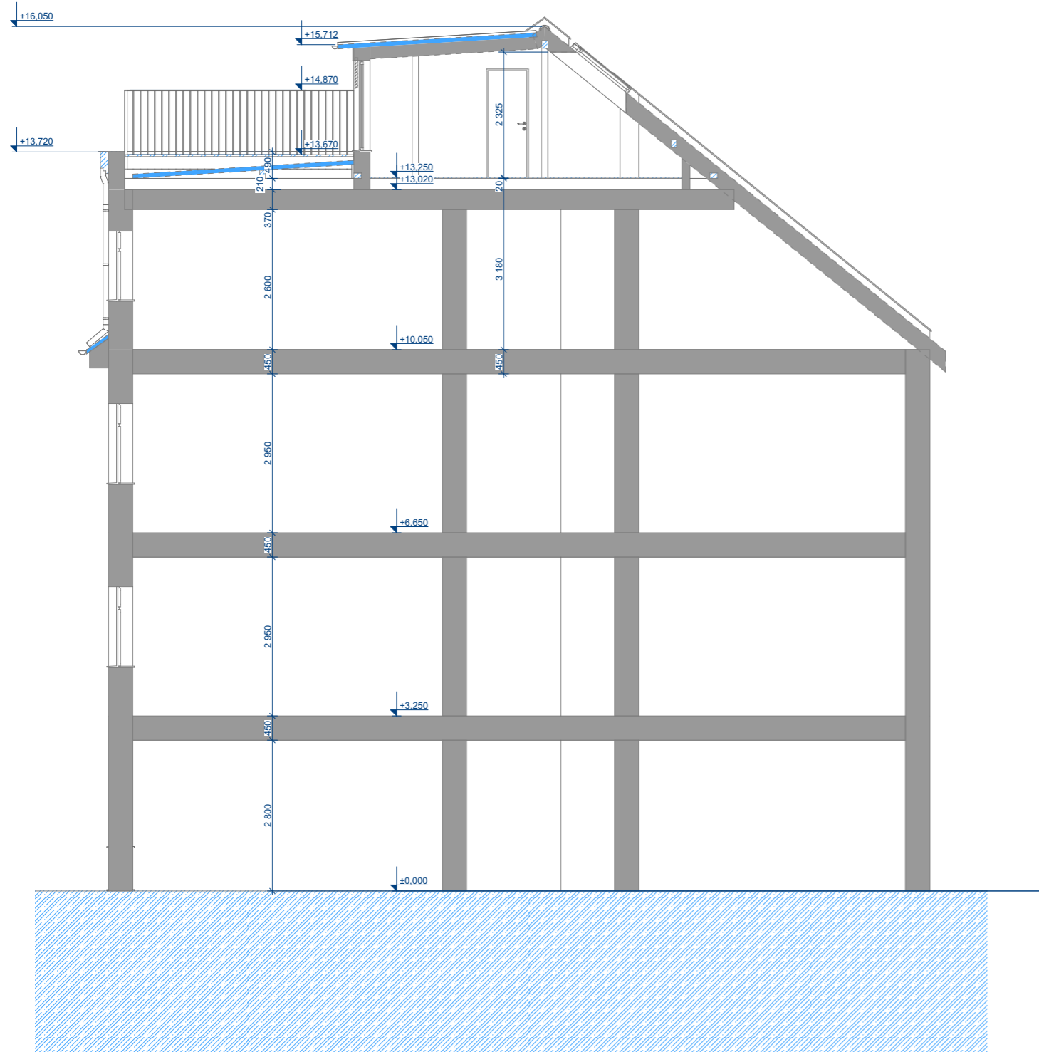
příčný řez A1, M. 1: 100
