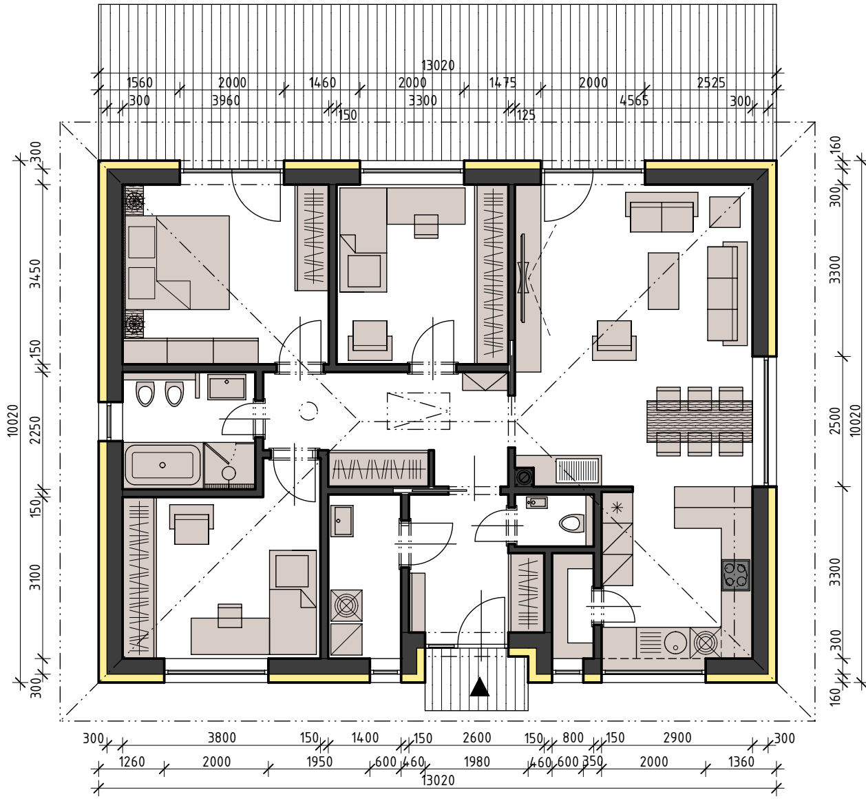
PÔDORYS PRÍZEMIA - 1.NP
