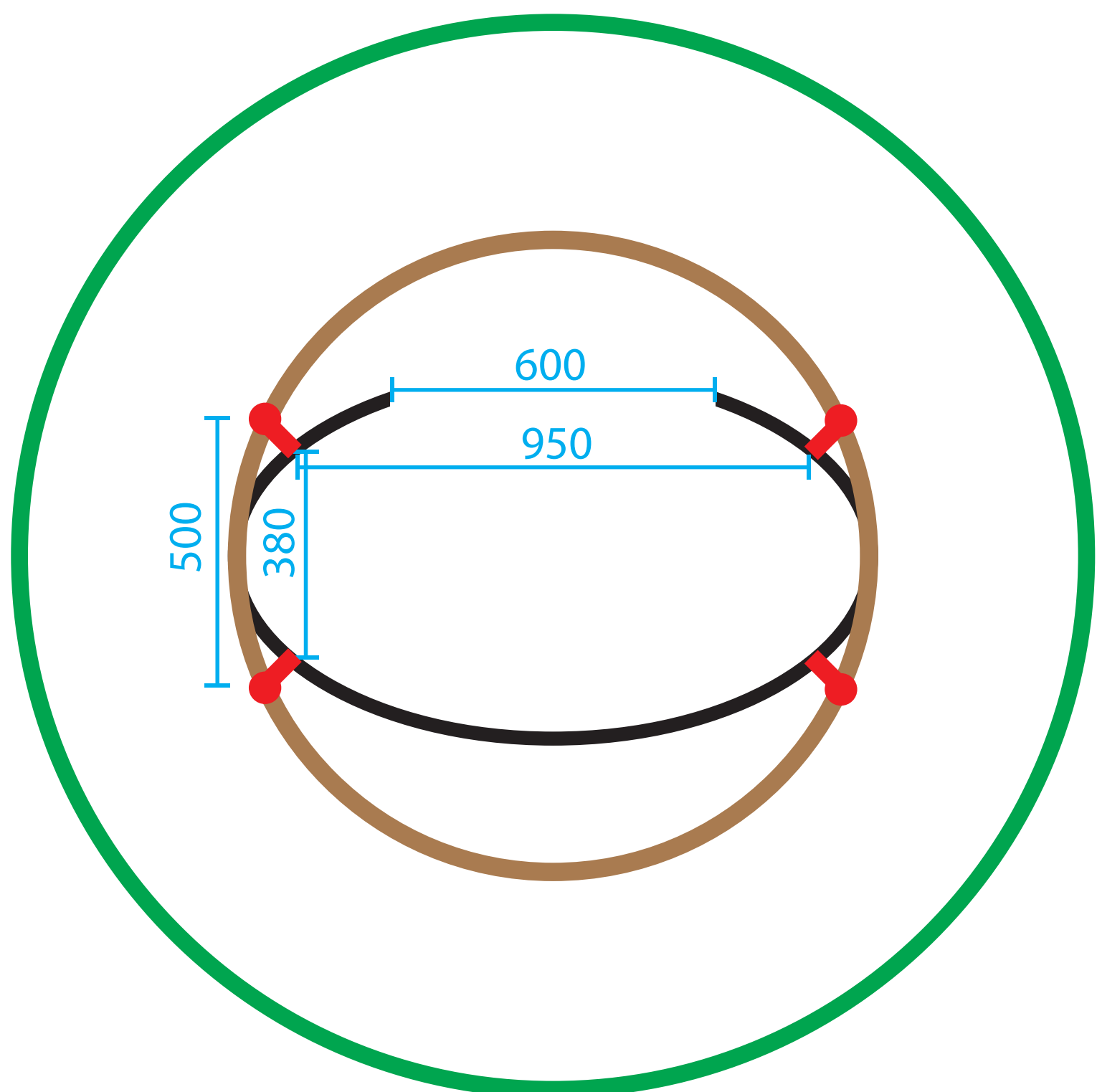
PŮDORYS
