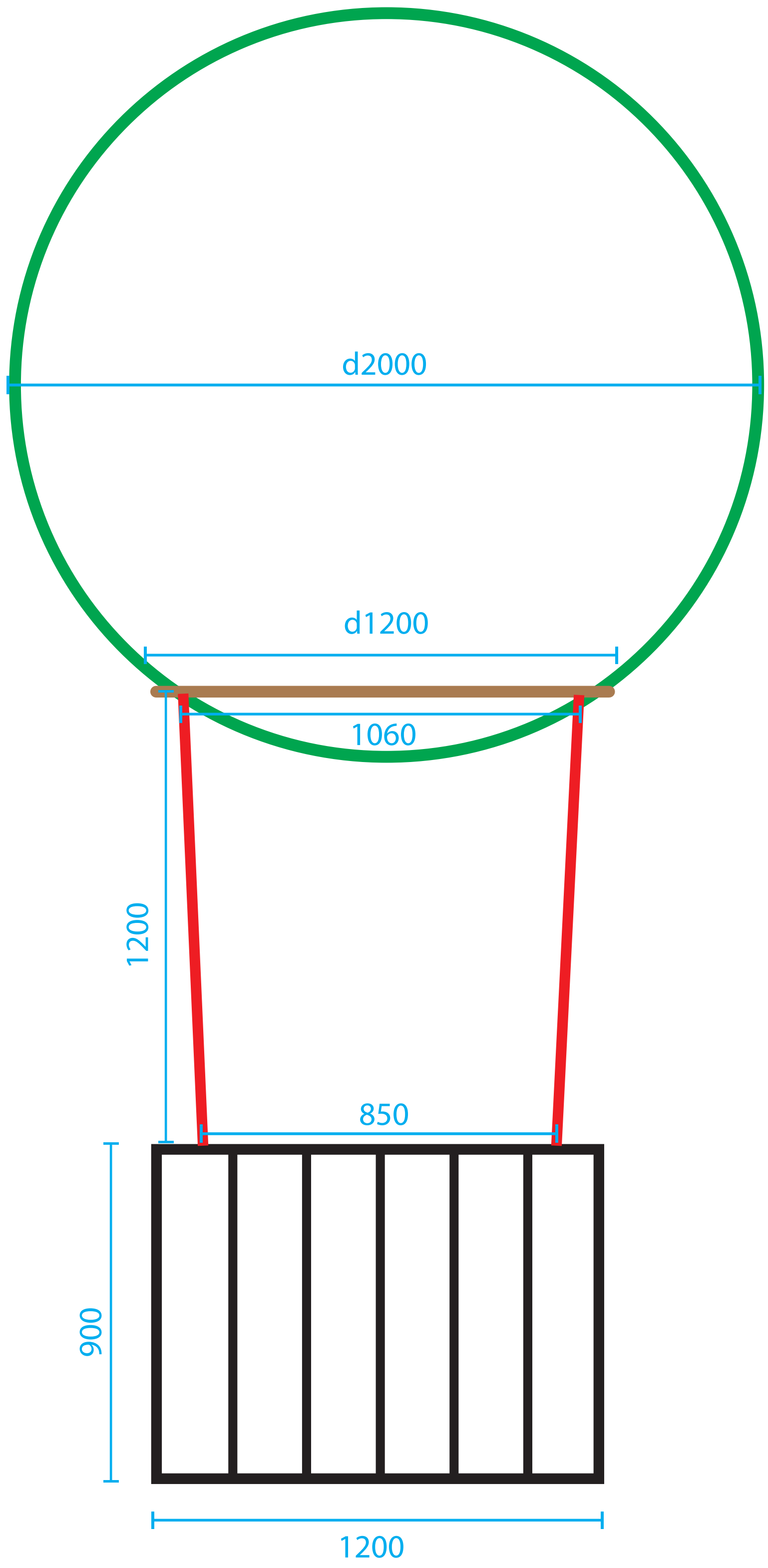
NÁRYS
