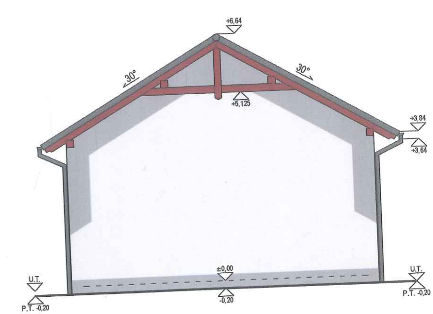
POHLED ZÁPADNÍ
