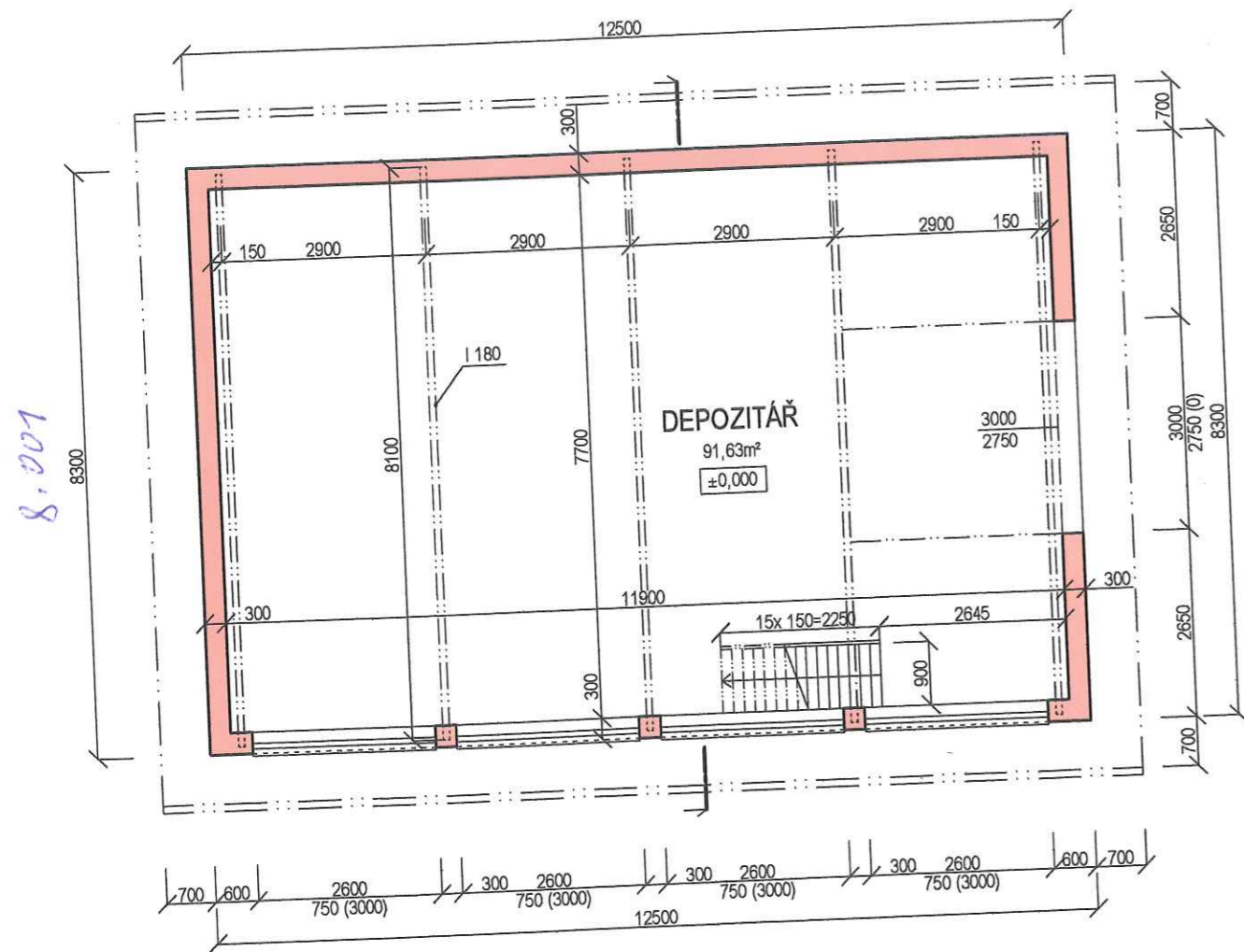
PŮDORYS
