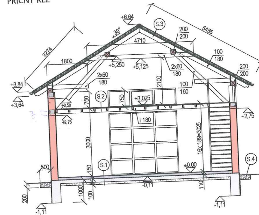
PŘÍČNÝ ŘEZ
