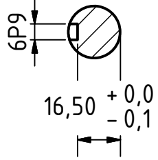
B-B ( 1 : 2 )
