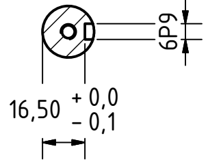
C-C ( 1 : 2 )
